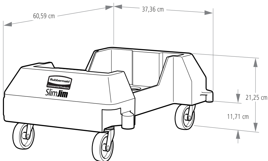
Socle d'enchaînement en résine
