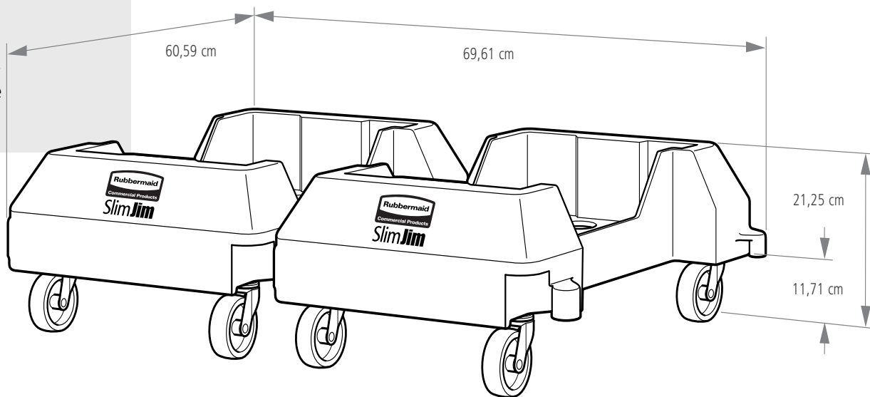
Socle d'enchaînement en résine
