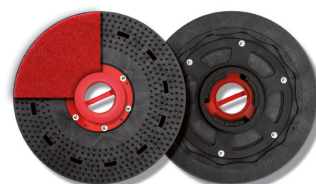
Plateau Padloc support disque Ø406mm réf.606401
